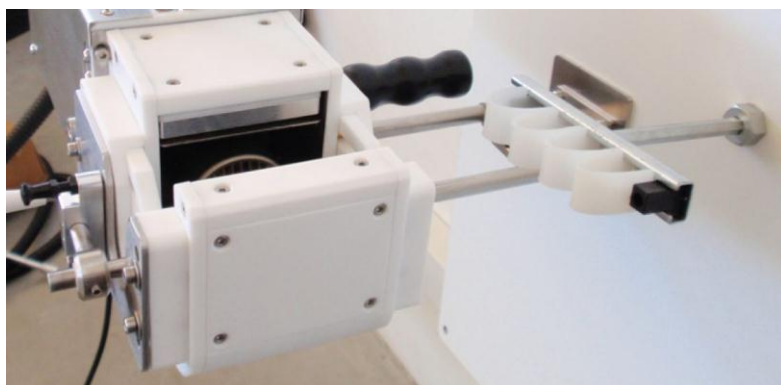
Fixation parallèle au panneau
